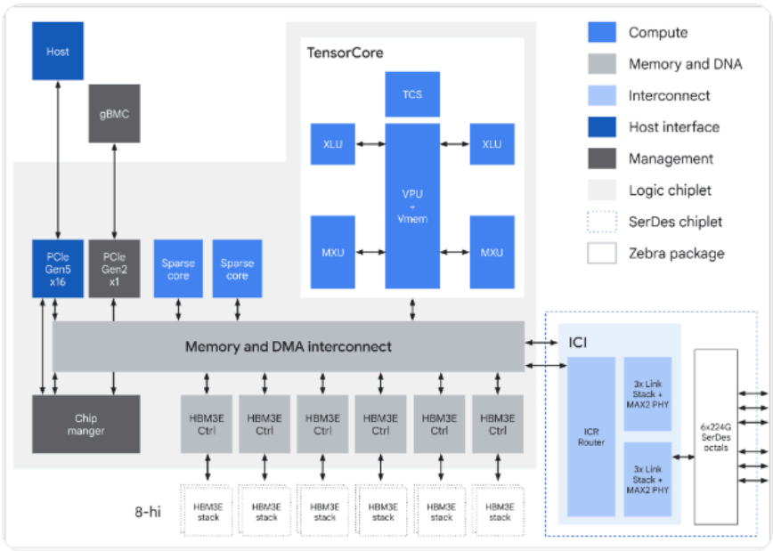
图1: TPU 8t ASIC 框图
